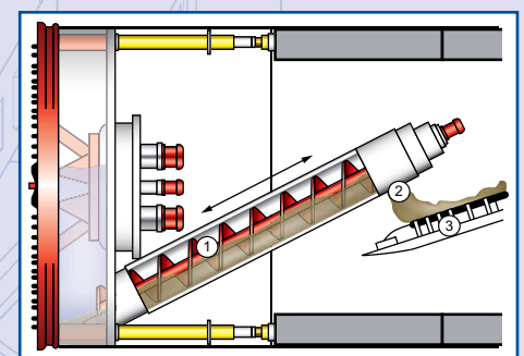
Grafik Funktionsprinzip der Förderschnecke im Schild einer EPB-Tunnelbohrmaschine (© Herrenknecht AG, Schwanau)
