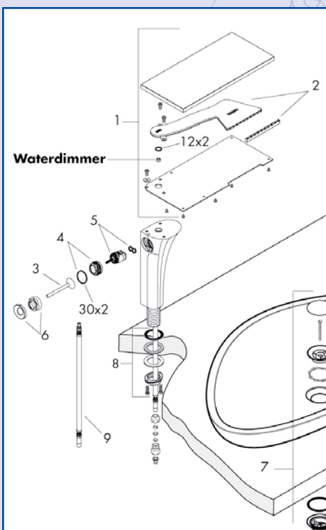
Explosionszeichnung eines Waschtischmischers (© Hansgrohe AG, Schiltach)
